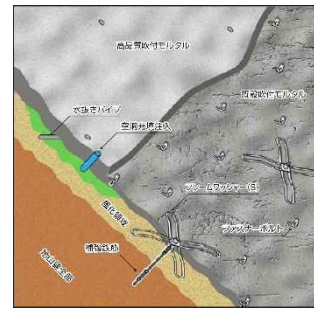
トーコンプラス工法 構造概略図(S、SG、L、LG タイプ)
