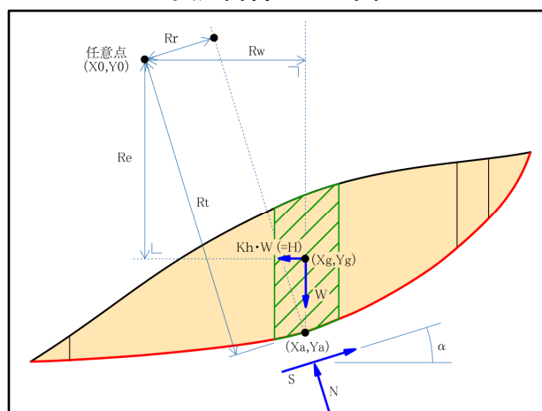
安定計算モデル図
