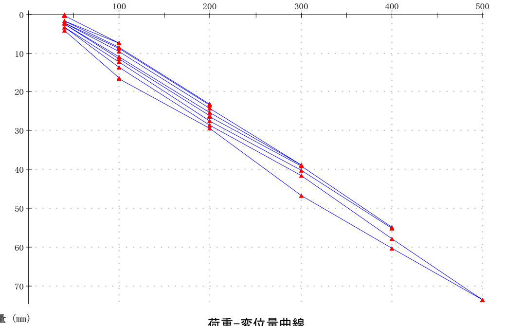
荷重-変位量曲線
