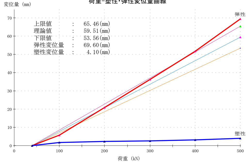
荷重-塑性・弾性変位量曲線
