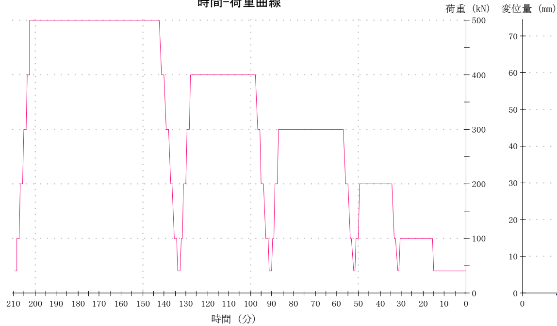
時間-荷重曲線
