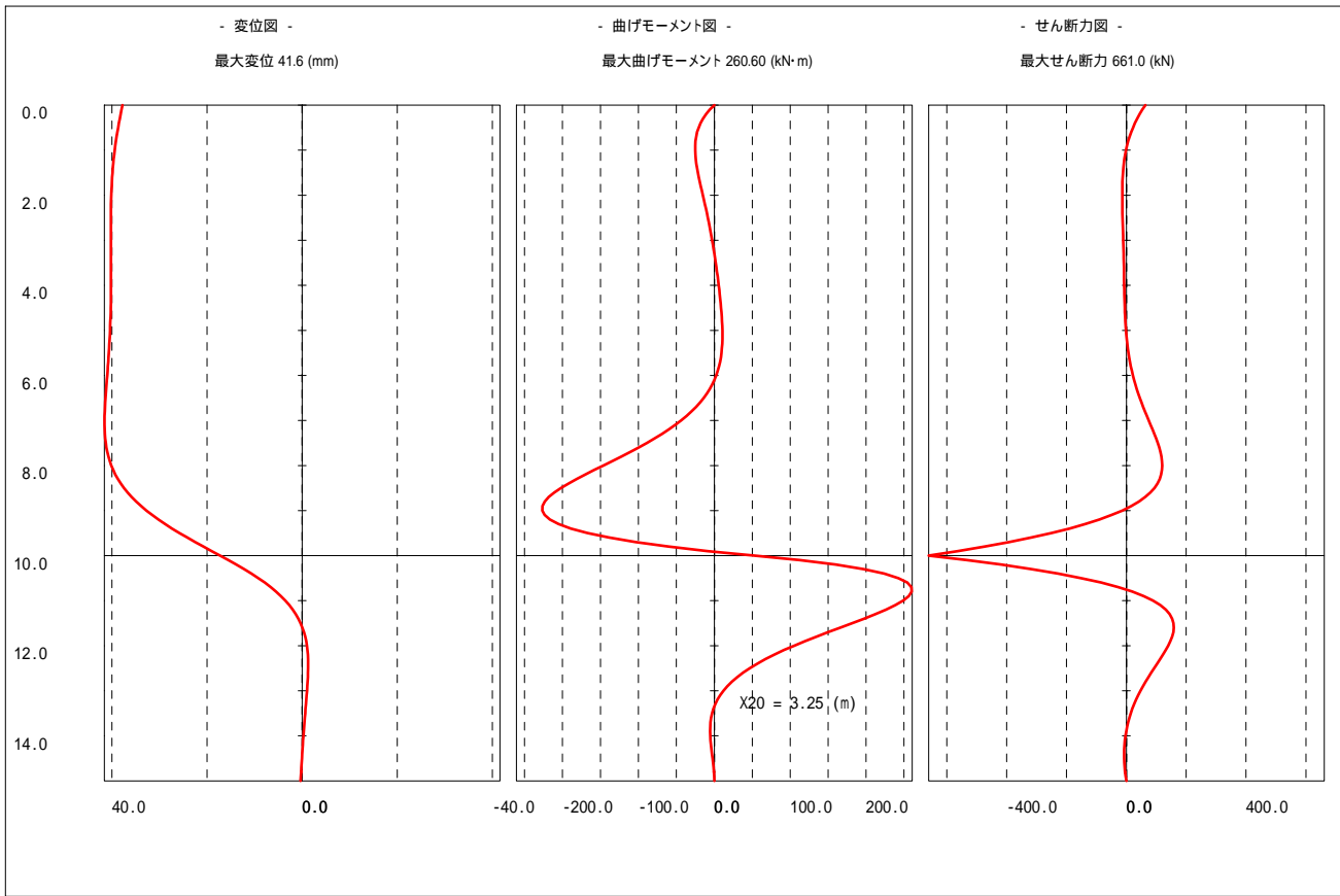
変位 - 曲げモーメント - せん断力
